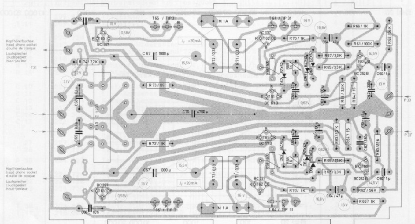
Fig. 5 Ätzsaltplatte des Endverstärkers 227 587 (Leiterseite)
