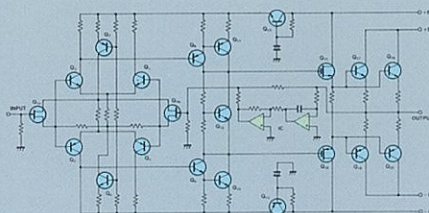
Abb. 1 Leistungsverstärker-Teil
