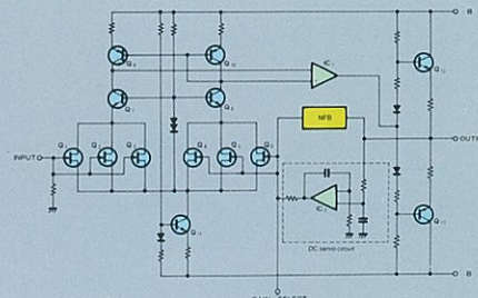
Abb. 2 Entzerrerverstärker-Teil
