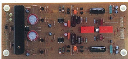
• Leiterplatte des hochverstärkenden Entzerrerverstärkers
